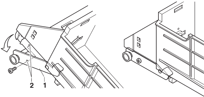
Fig. 32 1. Leva vassoi reclinabili 2. Fori bloccaggio leva (vassoi orizzontali)
